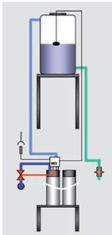
Instalacja do dejonizacji wody
